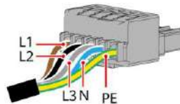
Klemme auf Wechselrichterseite (dreiphasig)
